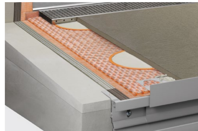
Свободная укладка на Schlüter-KERDI и Schlüter-TROBA-PLUS 8G
