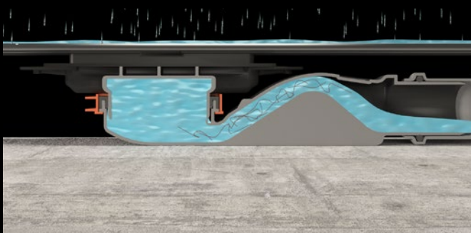
Эффект самоочистки благодаря высокой скорости потока
