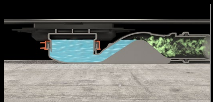
Постоянный сифонный затвор благодаря волнообразной форме
