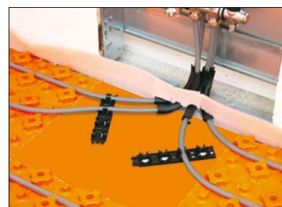
11 Verteilerbereich – Rohrklemmleisten Schlüter-BEKOTEC-BTZRKL zur Rohrführung nach Bedarf aufkleben.
