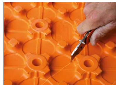
8 b Verarbeiten der Estrichnoppenplatte – Schneiden zwischen den Noppen: mit scharfem Messer/ Cutter anschneiden ... und brechen.
